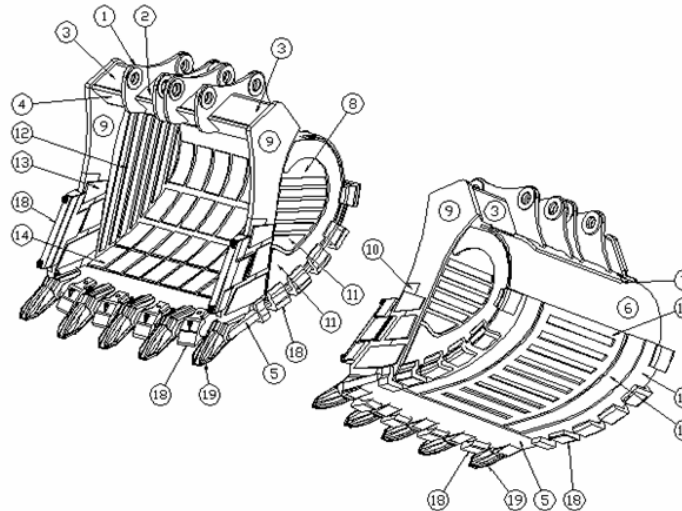
КОВШ
